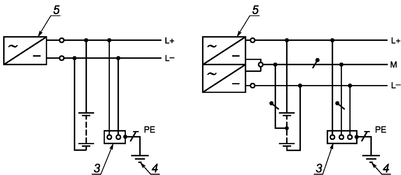
б) постоянного тока
