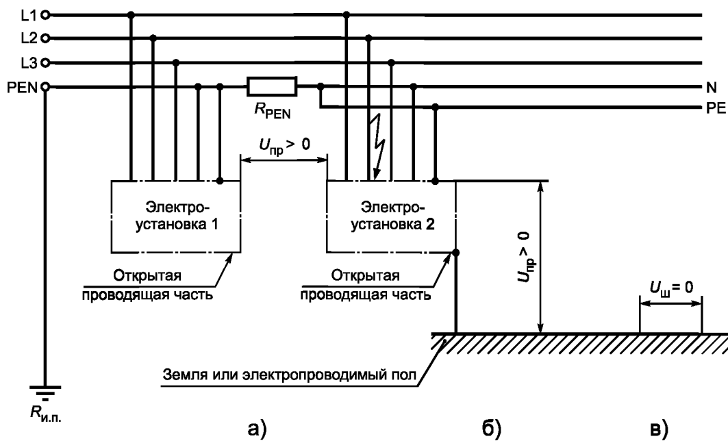
Рисунок Г.8 — Сеть TN-C-S с однофазным замыканием на корпус после точки разделения PEN-проводника на N- и PE-проводники
