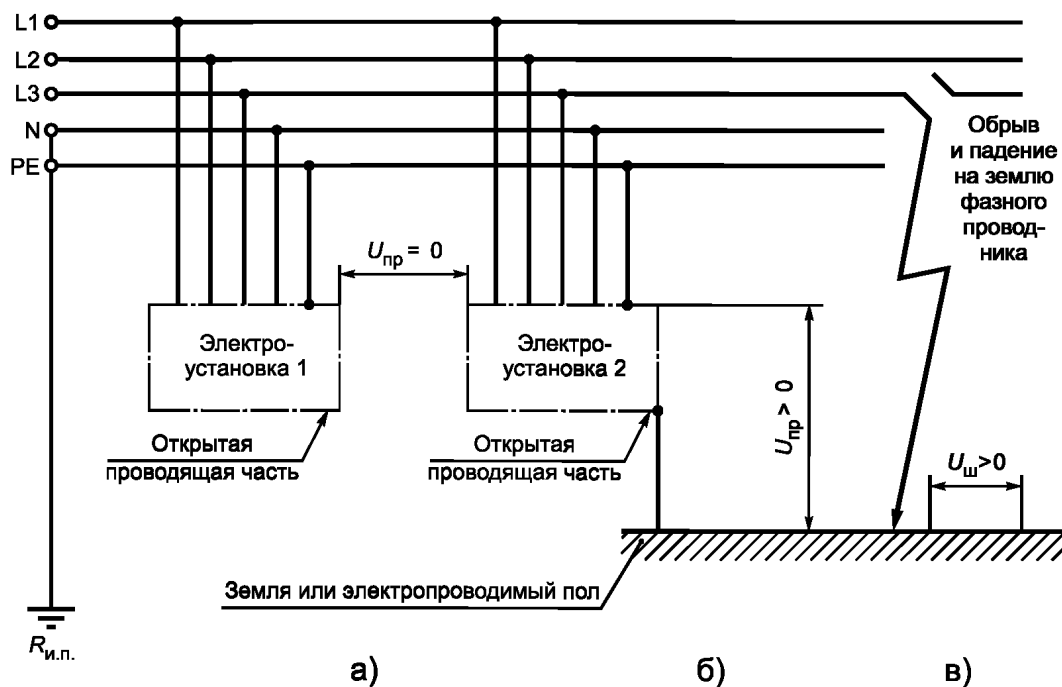
Рисунок Г.5 — Сеть TN-S с замыканием на землю, например с оборванным и упавшим на землю фазным проводом
