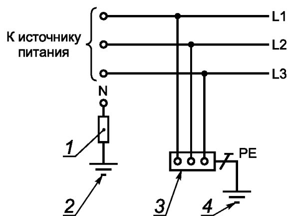
а) переменного тока
