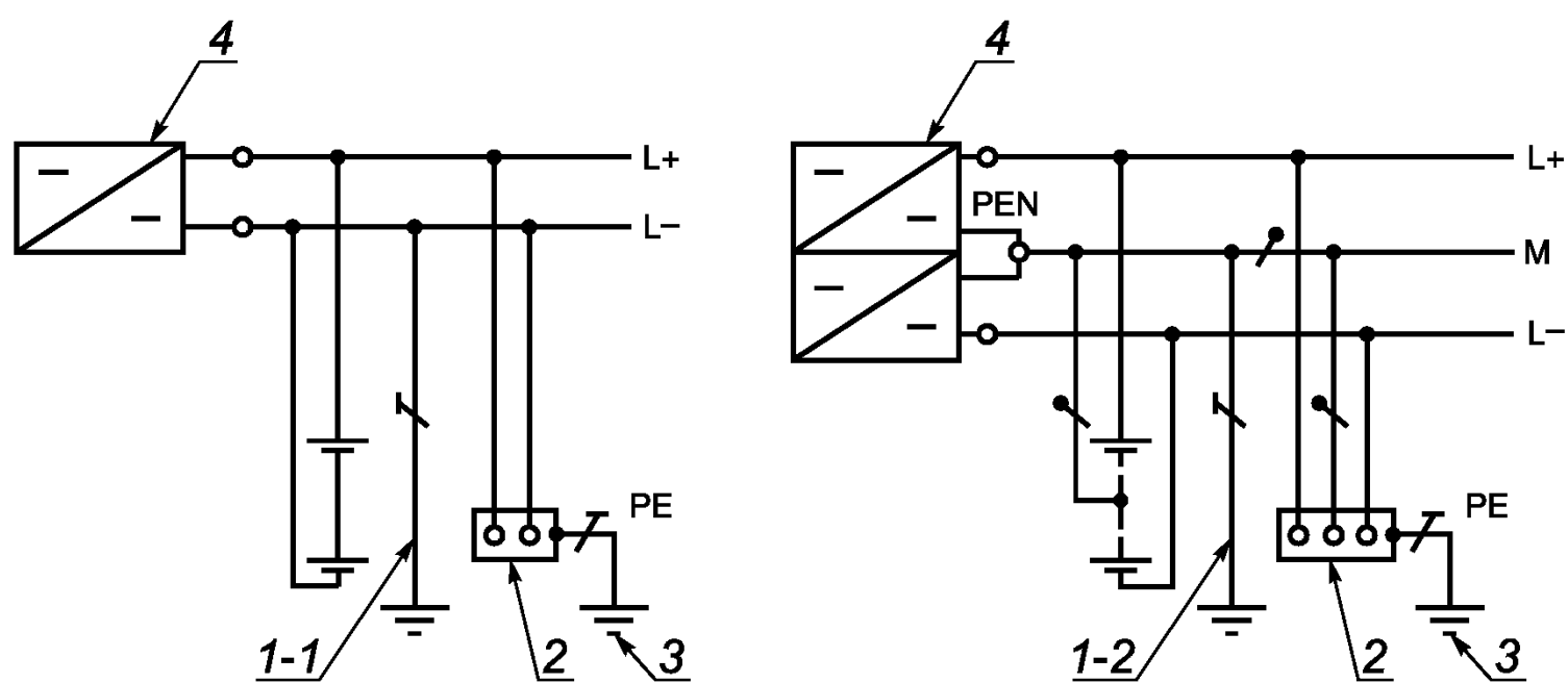
б) постоянного тока
