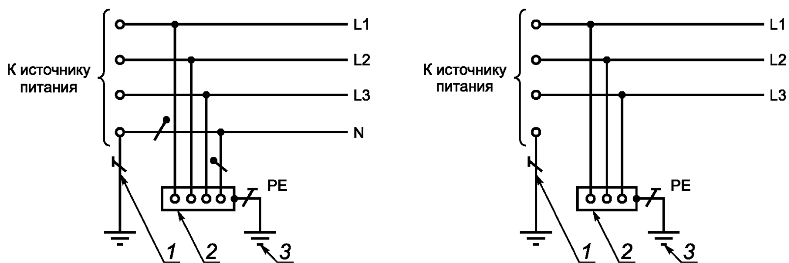
а) переменного тока
