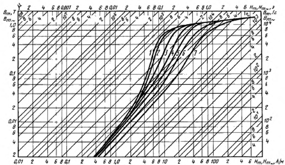
Кривые намагничивания сплава марки 50Н толщиной 0,1 мм для частот:
