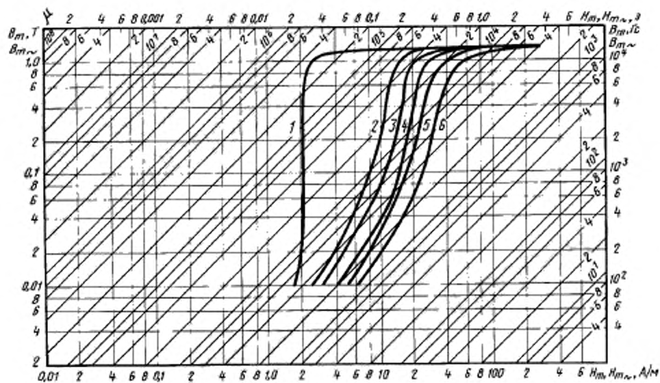
Кривые намагничивания сплава марки 40НХМП толщиной 0,05 мм для частот: 1 — 0 Гц; 2 — 400 Гц; 3 — 1000 Гц; 4 — 2000 Гц; 5 — 4000 Гц; 6 — 10000 Гц
