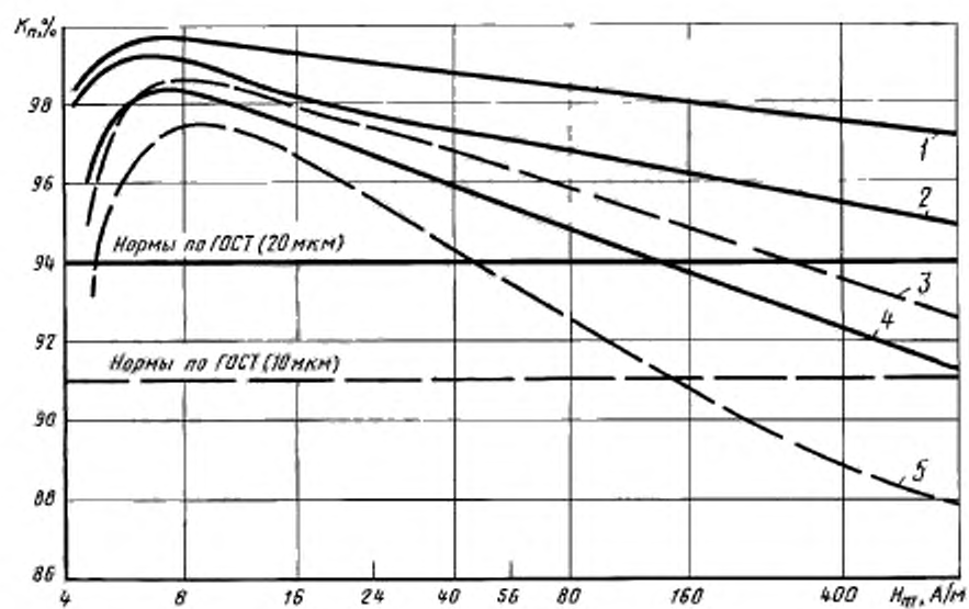
Зависимость коэффициента прямоугольности K_n от напряженности намагничивающего поля для сплава 50НП с разными значениями прямоугольности 1; 2; 3 — толщина 0,02 мм; 4; 5 — толщина 0,01 мм
