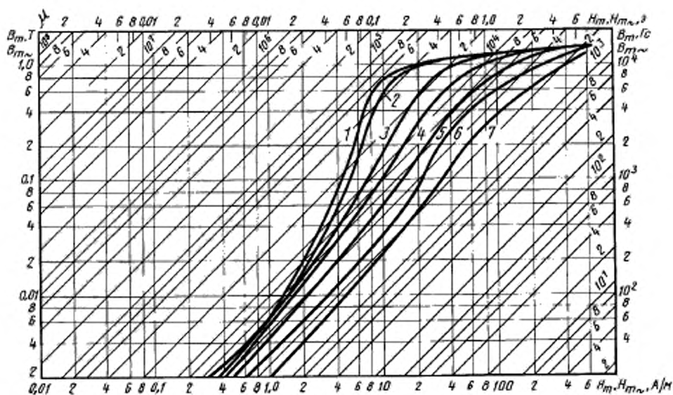
Кривые намагничивания сплава марки 50Н толщиной 0,2 мм для частот:
