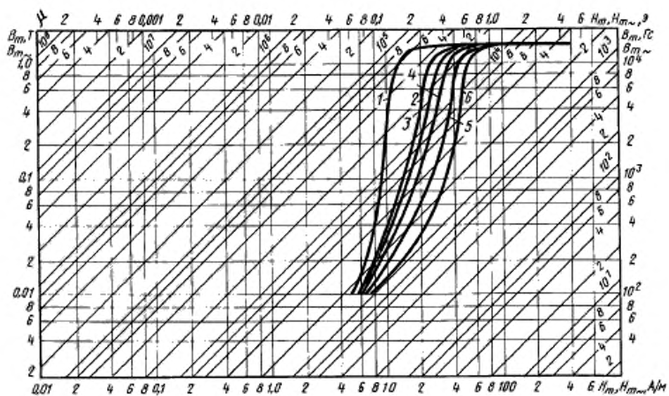
Кривые намагничивания сплава марки 50НП толщиной 0,05 мм для частот: 1 — 0 Гц; 2 — 400 Гц; 3 — 1000 Гц; 4 — 2000 Гц; 5 — 4000 Гц; 6 — 10000 Гц
