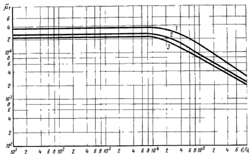
Зависимость \tilde{\mu}_1 от частоты для сплавов в лентах толщиной 0,02 мм марок: 1 — 83НФ; 2 — 80НХС; 3 — 79НМ
