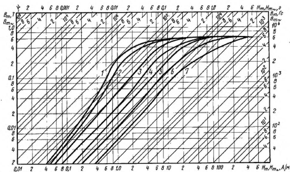
Кривые намагничивания сплава марки 80НХС толщиной 0,2 мм для частот: 1 — 0 Гц; 2 — 50 Гц; 3 — 400 Гц; 4 — 1000 Гц; 5 — 2000 Гц; 6 — 4000 Гц; 7 — 10000 Гц
