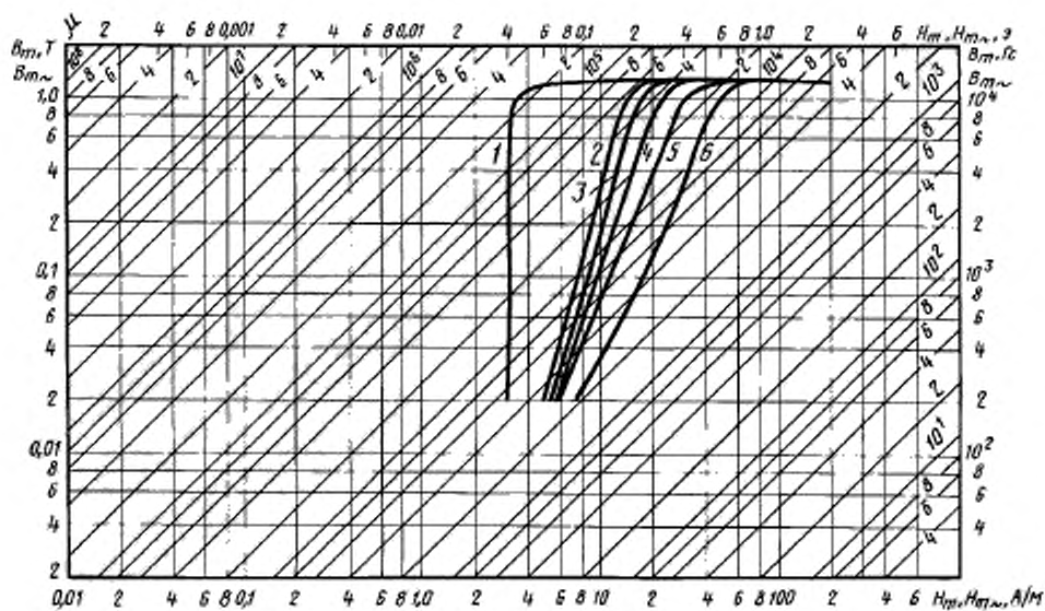
Кривые намагничивания сплава марки 35НХСП толщиной 0,05 мм для частот: 1 — 0 Гц; 2 — 400 Гц; 3 — 1000 Гц; 4 — 2000 Гц; 5 — 4000 Гц; 6 — 10000 Гц
