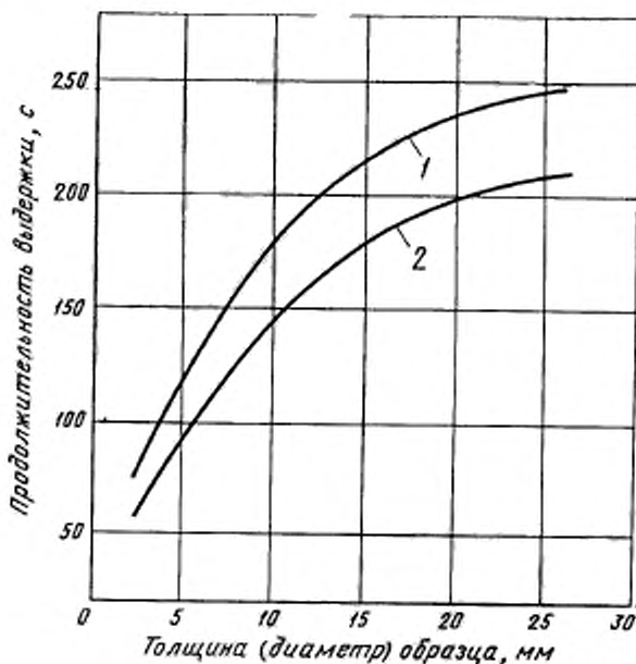
1 — для прямоугольных образцов; 2 — для круглых образцов
