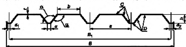
B_1 — монтажная ширина профиля; B — общая ширина; h — высота гофра; t — толщина профиля; s — шаг гофров; a и b — ширина полки профиля (в ряде случаев a = b ); a_1 и a_2 — ширина крайних полков гофров профиля, C — наружная (лицевая) сторона профиля; D — обратная сторона профиля
