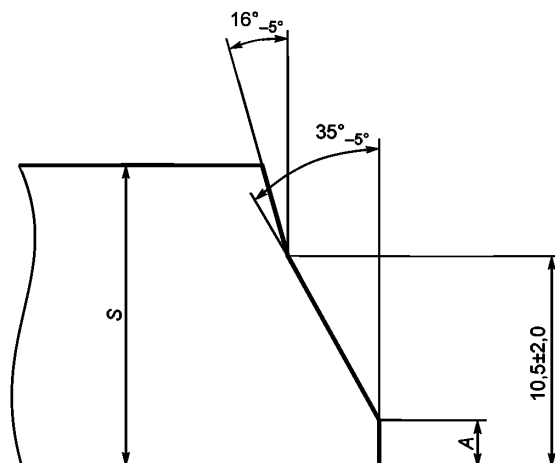
A — ширина торцевого притупления, S — толщина стенки
